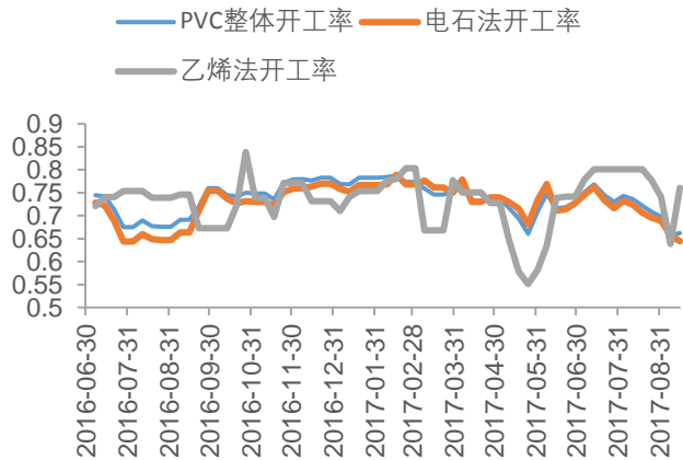
图 6：PVC 装置开工率
