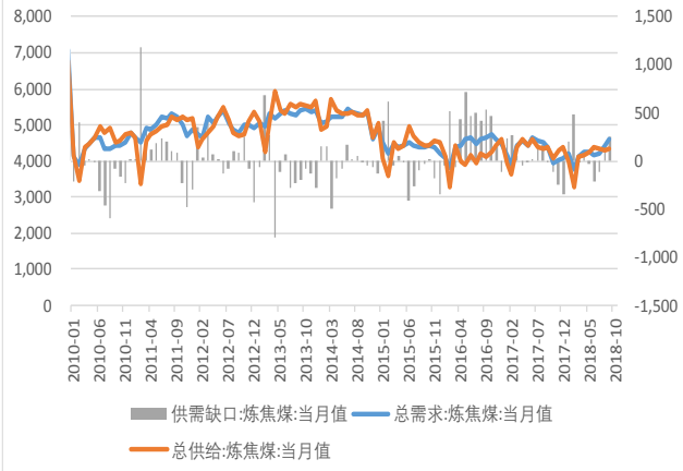
炼焦煤供需缺口
