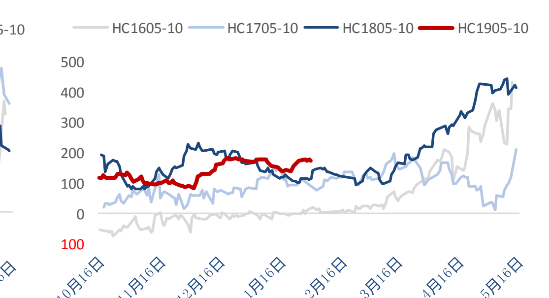
图14：热卷5-10价差
