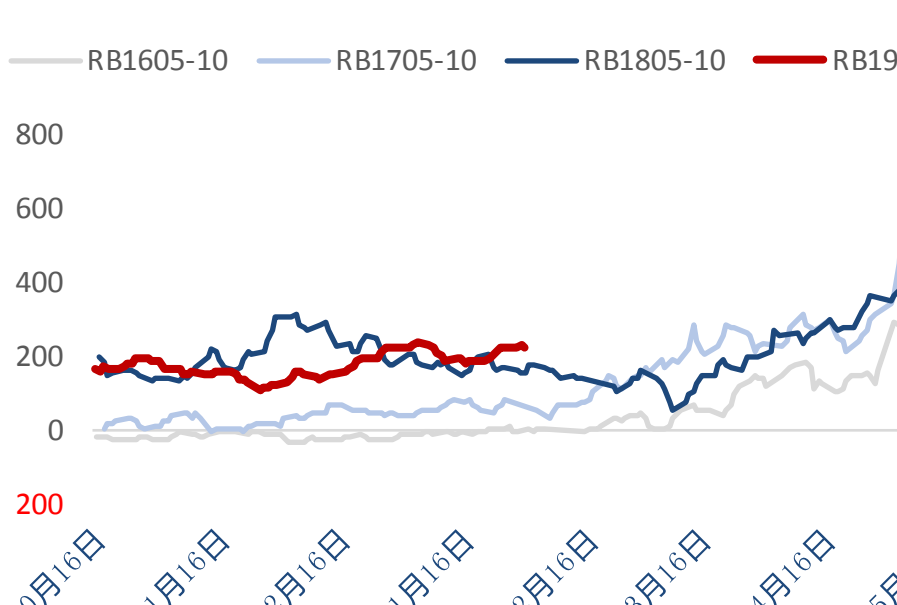
图13：螺卷5-10价差
