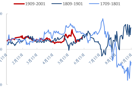
图9：焦炭9-1价差
