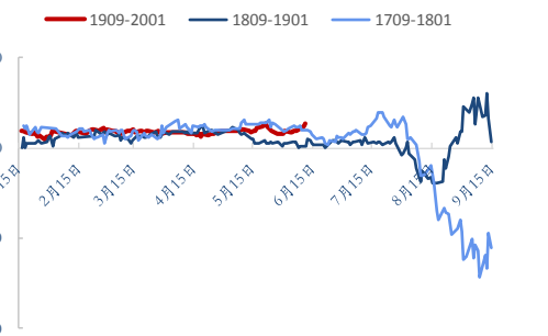
图10：焦煤9-1价差
