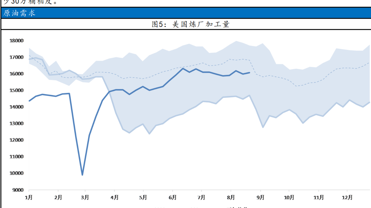
图5：美国炼厂加工量
